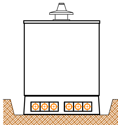
LATO DESTRO
