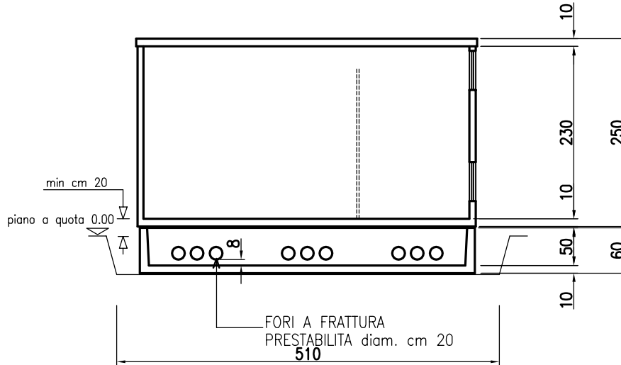
SEZIONE A-A
