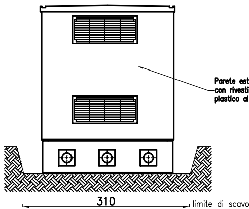
LATO SINISTRO
